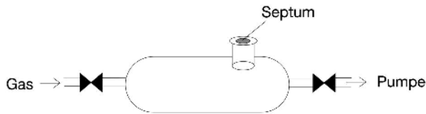
Abbildung 1.7 Gasmaus zur Probenahme von Gasen.
